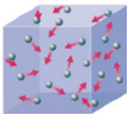
Слика 3.2. Движењето на честичките од гасот и нивните заемодејства ја сочинуваат внатрешната енергија на системот.
