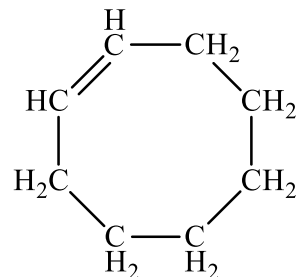
Циклооктен
