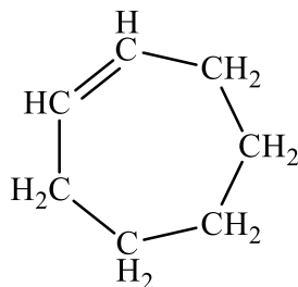
Циклохептен
