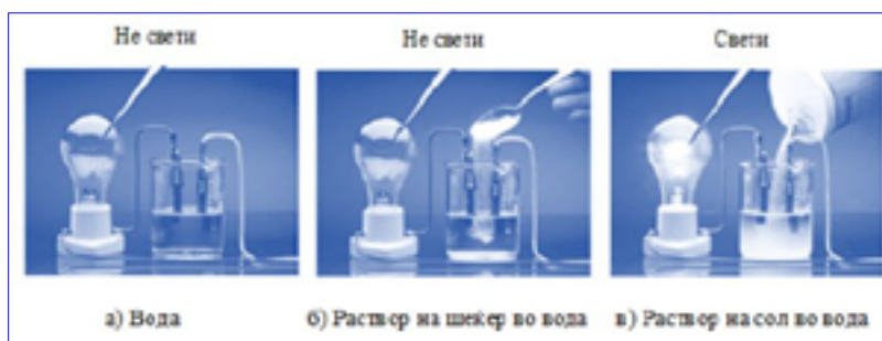
Слика 2.9. Сијаличката не свети кога електродите се вронети во чиста вода (а) и во раствор на шеќер во вода (б), но свети кога тие се вронети во раствор на сол во вода.
