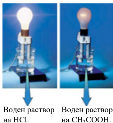
Слика 2.10. Сијаличката свети посилно кога електродите се вронети во раствор на \text{HCl} , отколку кога се вронети во раствор на \text{CH}_3\text{COOH} .
